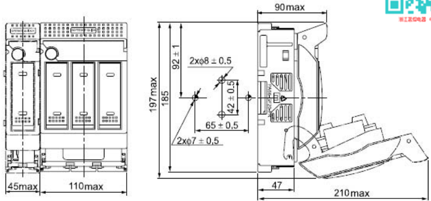
图 15.4 MRO.H1(DR1)-160 MRO.H1(DR1)-160/4
